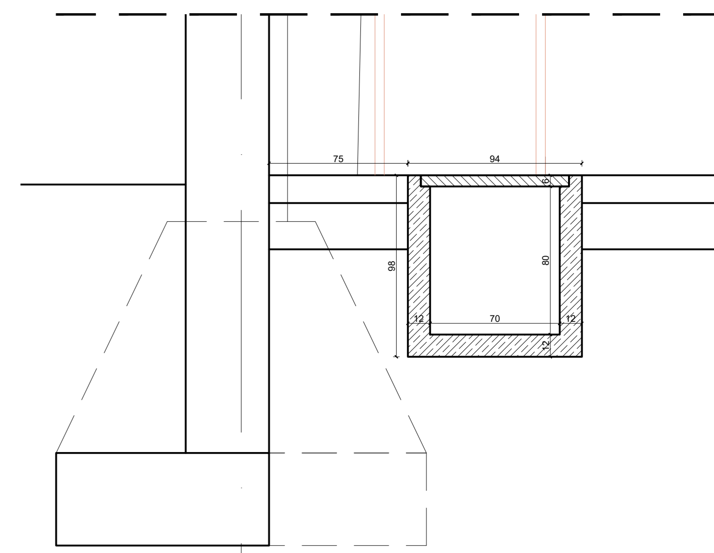
PRZEKRÓJ POPRZECZNY PRZEZ KANAŁ TECHNICZNY Skala 1:20
