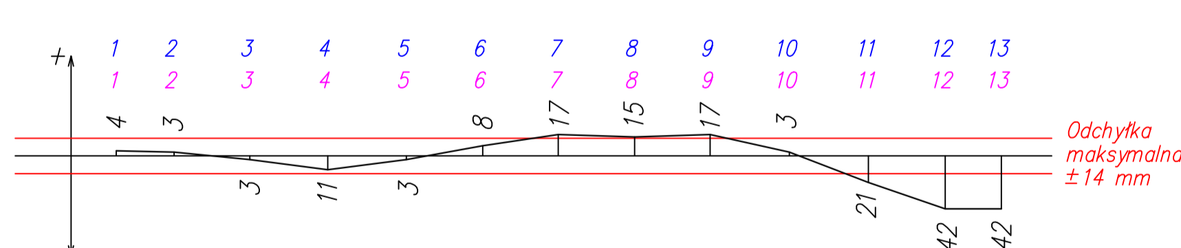
Wykres prostoliniowości szyny lewej [mm]
