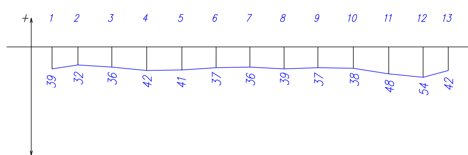
Wykres odkształceń pionowych szyny lewej [mm]
