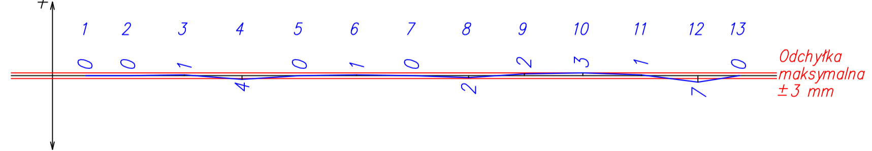
Wykres prostoliniowości szyny prawej [mm]
