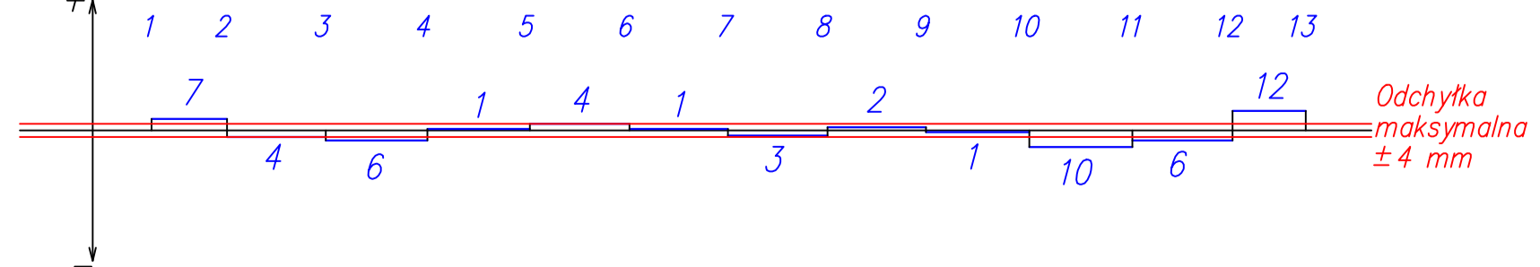
Wykres różnic wysokości nivelety szyny lewej [mm]
