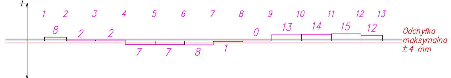
Wykres różnic wysokości nivelety szyny prawej [mm]
