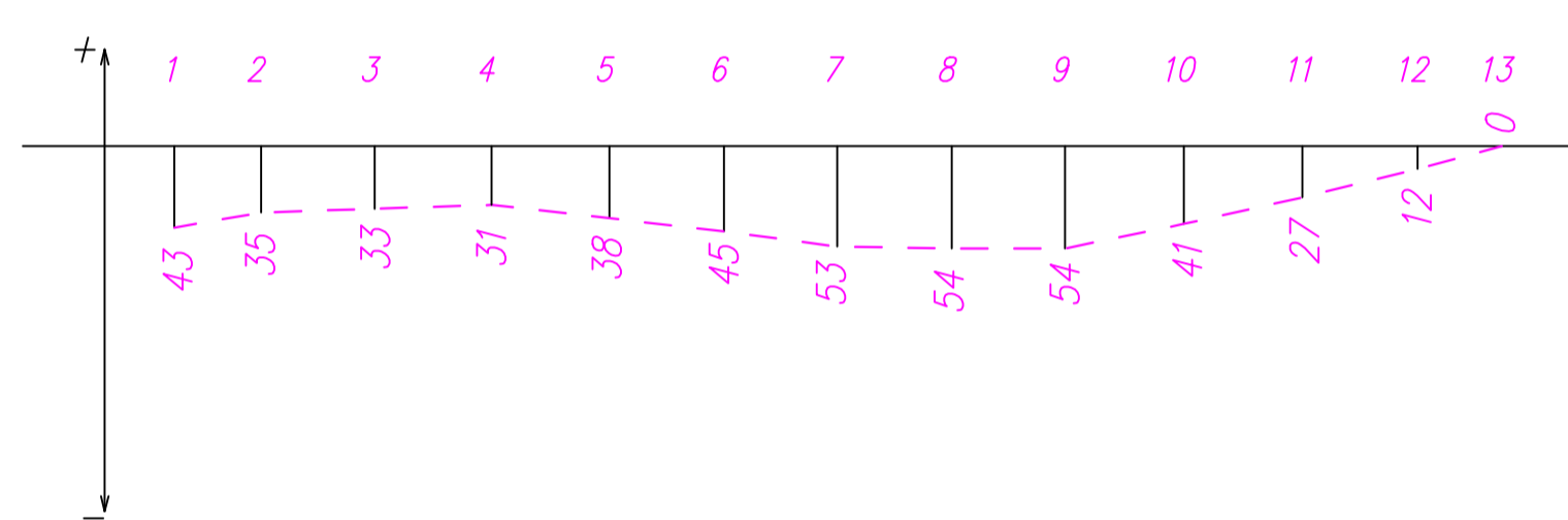
Wykres odkształceń pionowych szyny prawej [mm]
