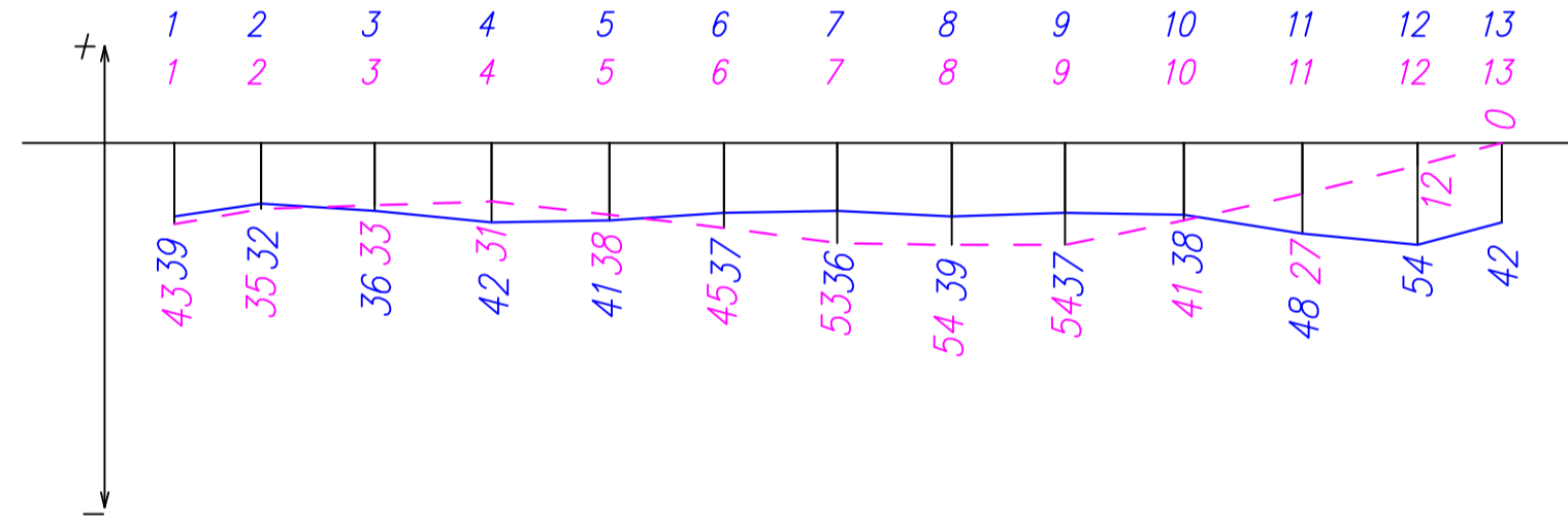
Wykres odkształceń pionowych szyny prawej [mm]
