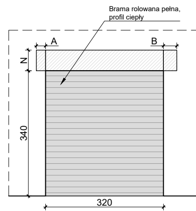
Brama B1 zewnętrzna rolowana (rozwiązanie alternatywne) Widok od strony pomieszczenia 01
