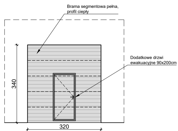
Brama B4 segmentowa z drzwiami Widok od strony pomieszczenia 13
