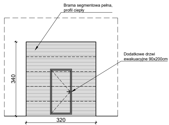
Brama B1 zewnętrzna segmentowa z drzwiami Widok od strony pomieszczenia 01
