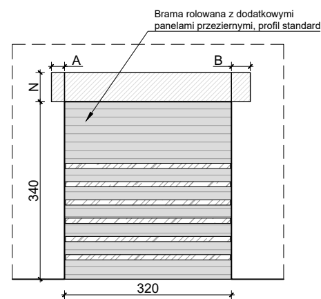
Brama B3 rolowana (rozwiązanie alternatywne) Widok od strony pomieszczenia 13
