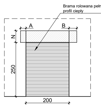
Brama B2 (rozwiązanie alternatywne) Widok od strony pomieszczenia 13
