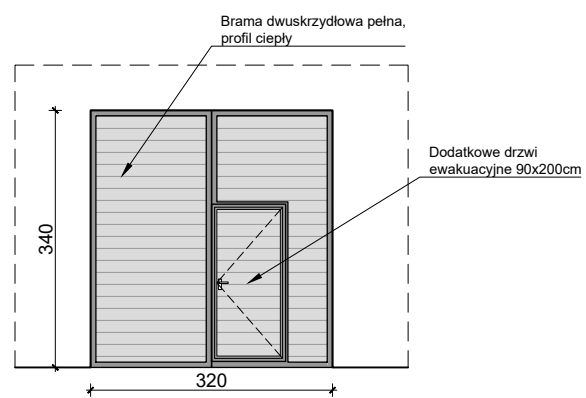
Brama B6 dwuskrzydłowa z drzwiami Widok od strony pomieszczenia 16
