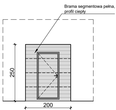
Brama B2 segmentowa z drzwiami Widok od strony pomieszczenia 13
