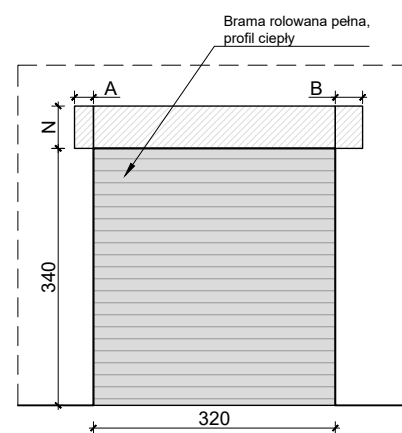
Brama B4 rolowana (rozwiązanie alternatywne) Widok od strony pomieszczenia 13
