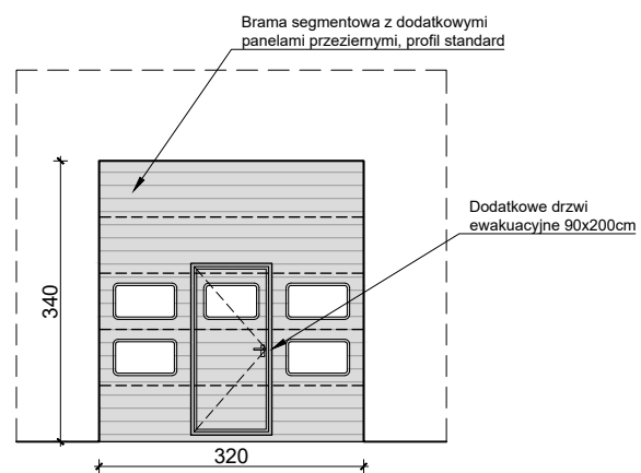
Brama B3 segmentowa z drzwiami Widok od strony pomieszczenia 13
