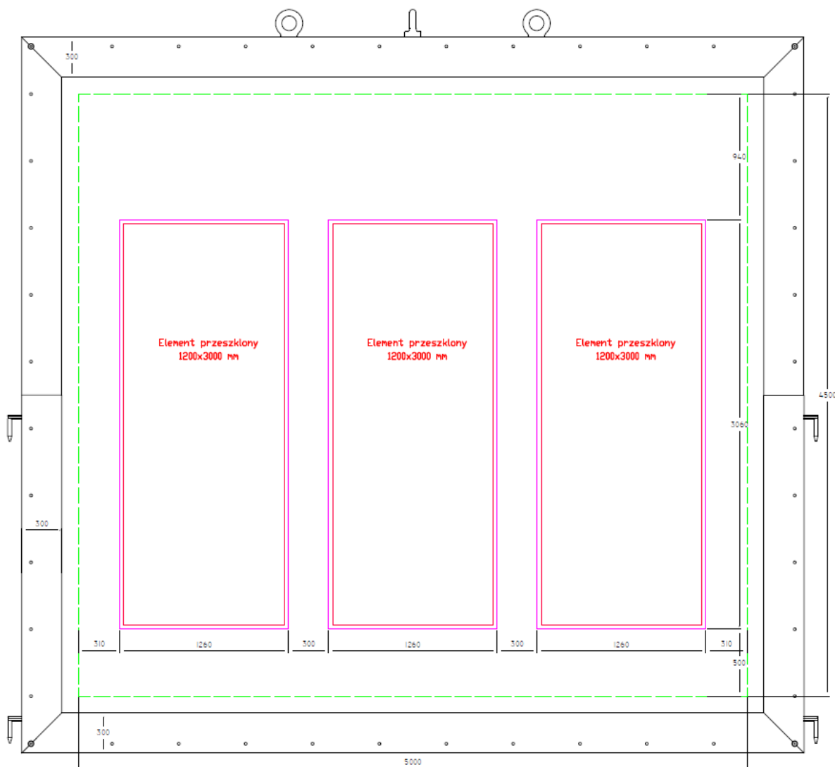
Rysunek – konstrukcja mocująca wymiary i położenie próbek
